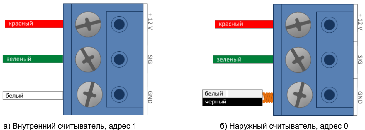
Рисунок 8. Подключение считывателя в режиме «карта + ПИН»
